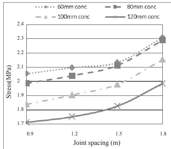
b.) Load case 2
