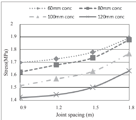
a.) Load case 1
